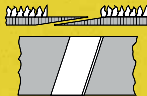
Forma 5 Slepeno s přesahem. Zóna zrna plně zbroušena. Použití na bruskách s plochou kontaktní botkou, umožňuje jemný přechod oblastí pásového spoje.
